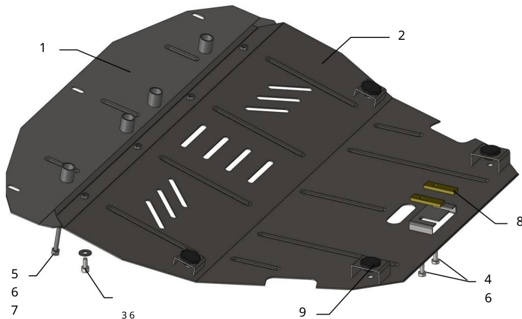
Schéma montáže ochrany klukovej skrine.
