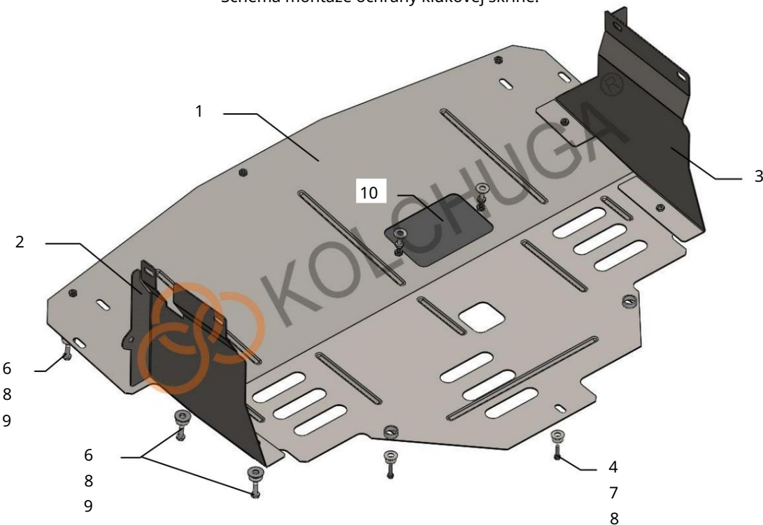
Schéma montáže ochrany klúčovej skrine.
