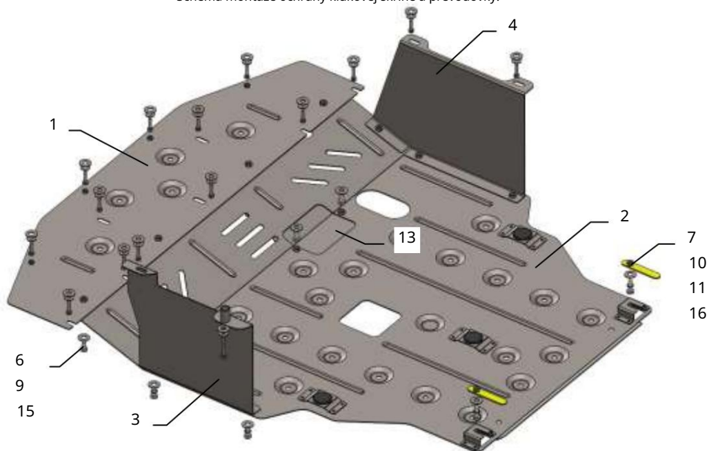
Schéma montáže ochrany kľúčovej skrine a prevodovky.
