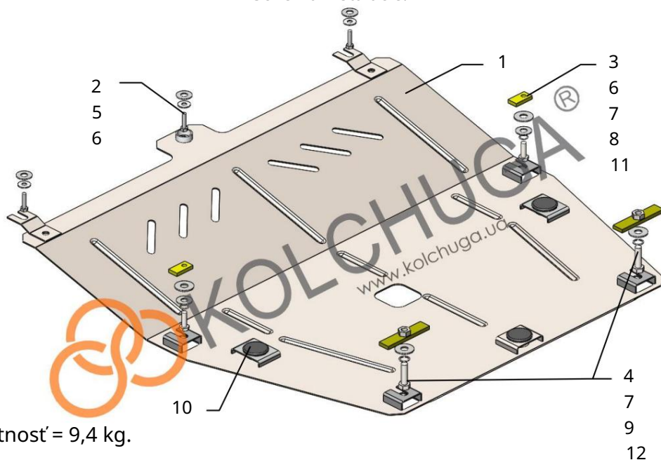
Schéma inštalácie.
