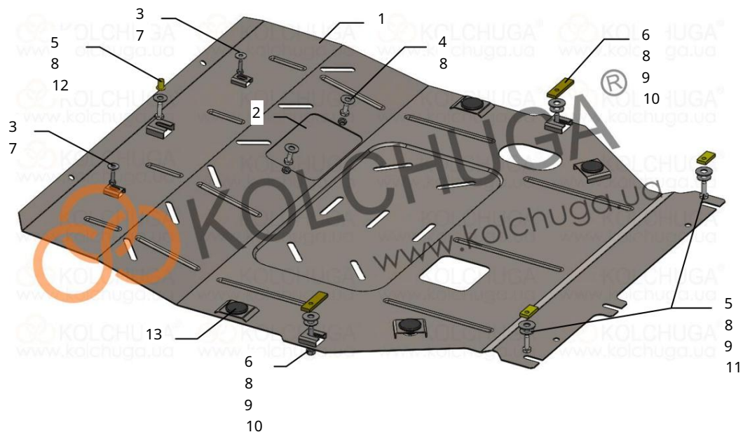
Schéma montáže ochrany motoru a převodovky
