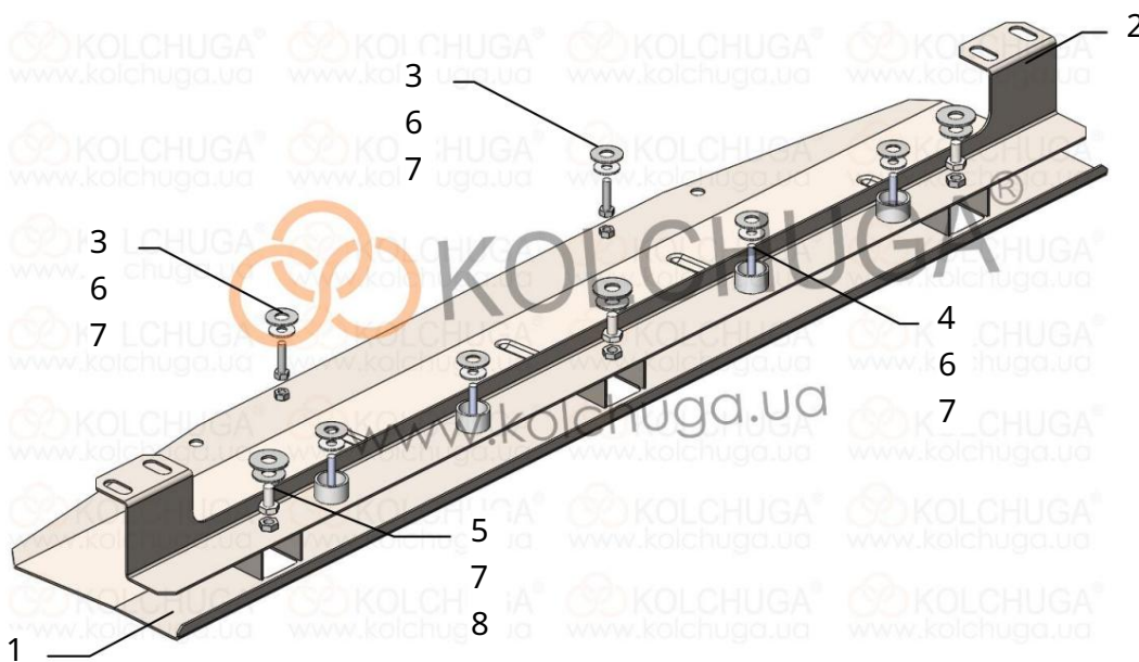
Schéma montáže ochrany chladiča
