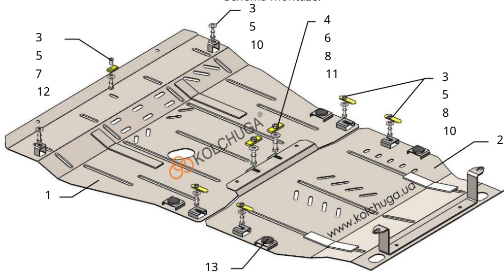
Schéma montáže.
