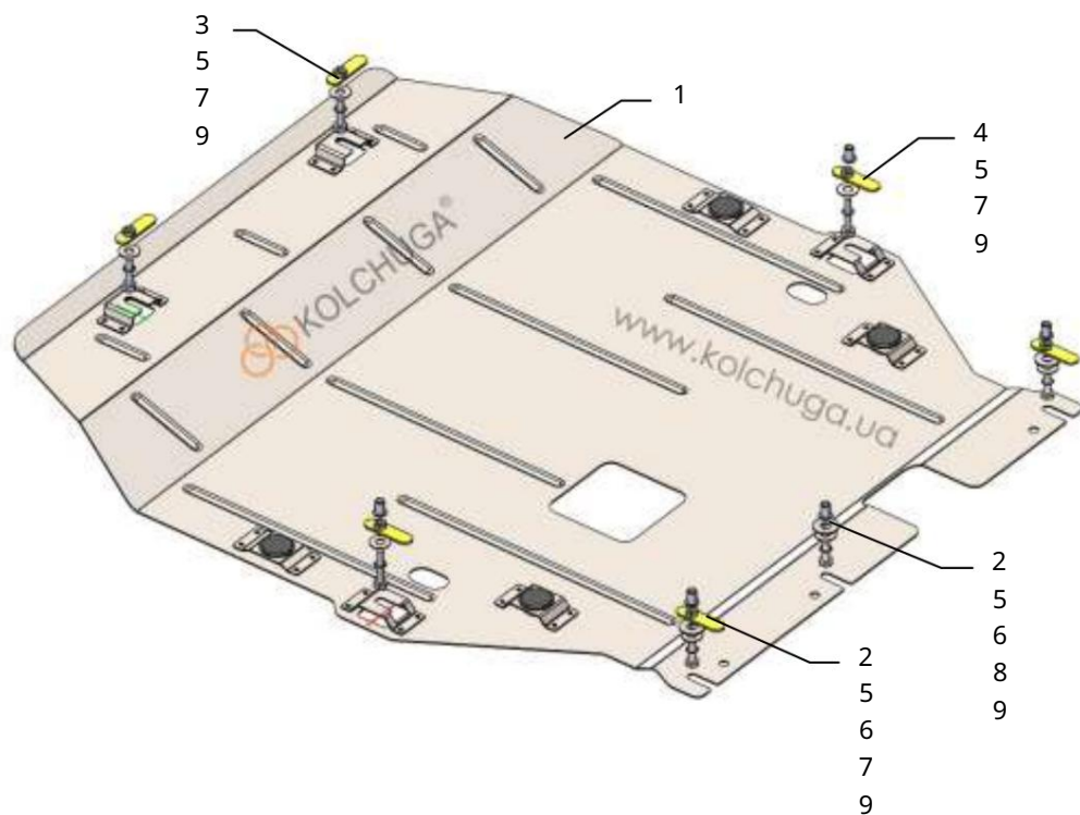
Schéma montáže ochrany motora a prevodovky
