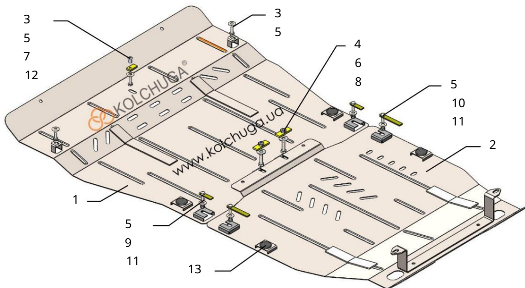
Schéma montáže.
