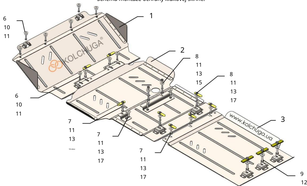
Schéma montáže ochrany kľúčovej skrine.
