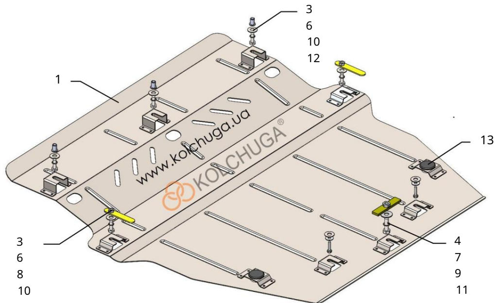
Schéma montáže.
