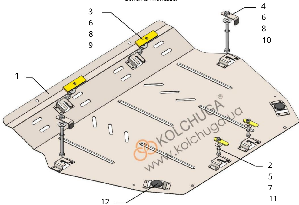
Schéma montáže.
