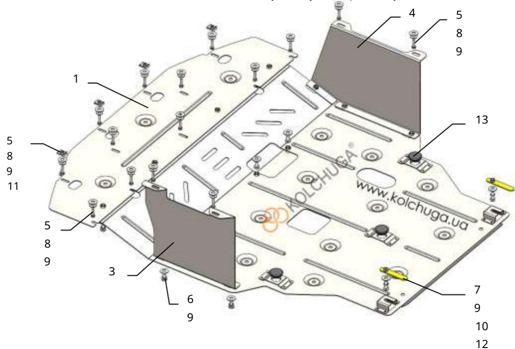
Schéma montáže ochrany klukovej skrine a prevodovky.
