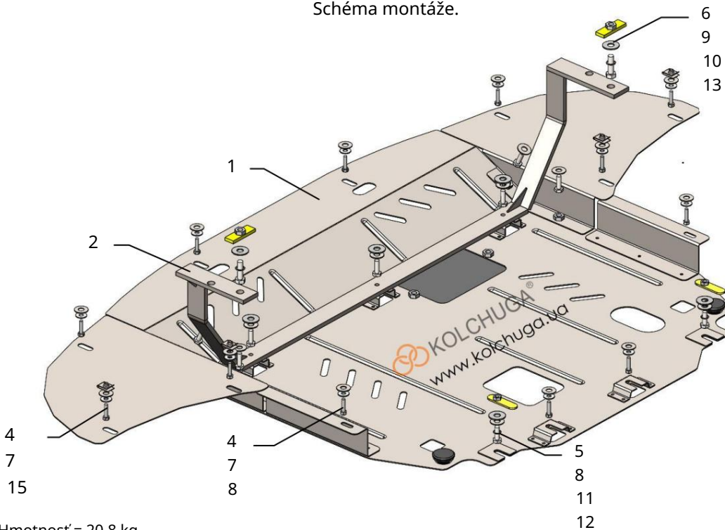
Schéma montáže.
