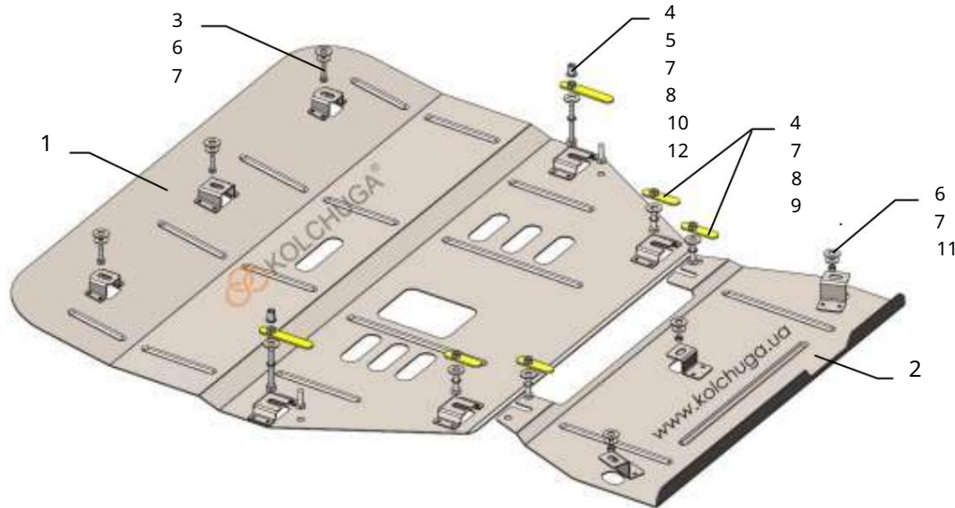
Schéma montáže.
