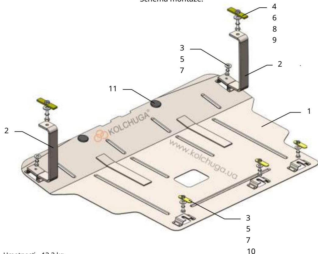
Schéma montáže.
