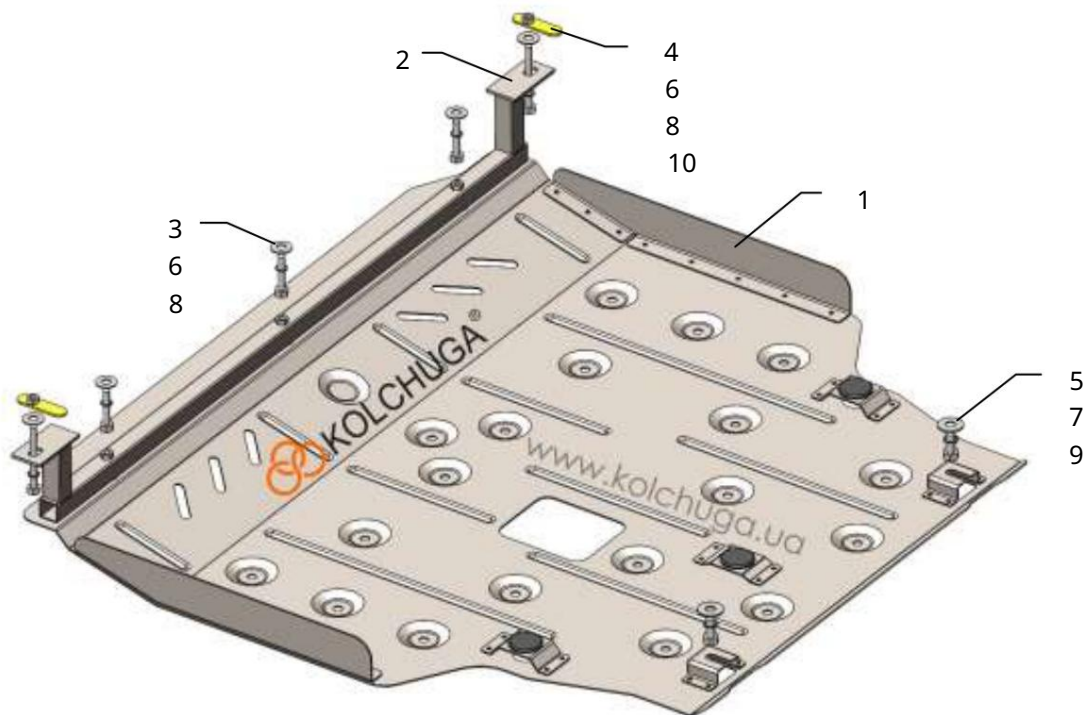
Schéma inštalácie.
