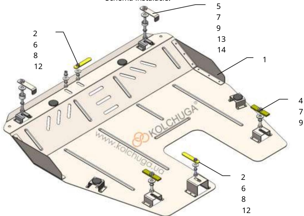
Schéma inštalácie.
