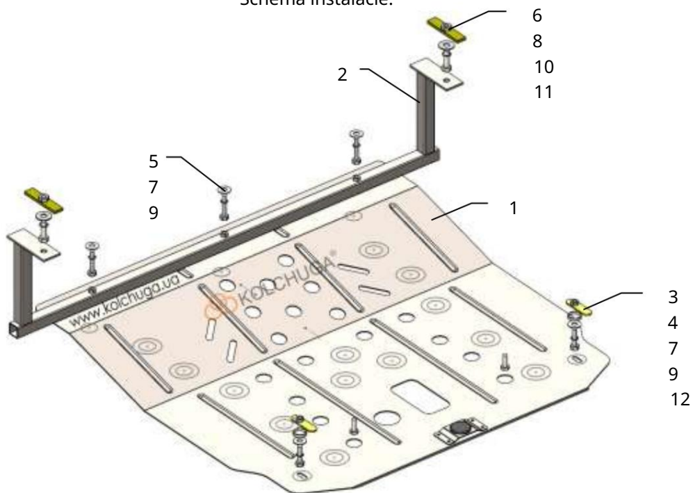
Schéma inštalácie.
