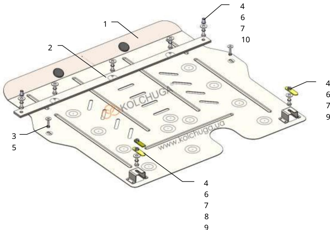
Schéma inštalácie.
