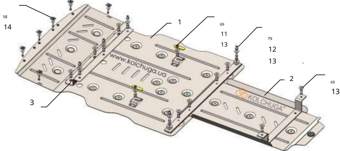
Schéma montáže.
