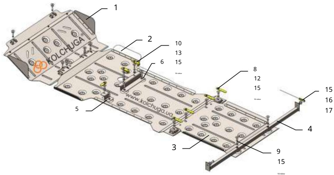
Schéma montáže ochrany klukovej skrine.
