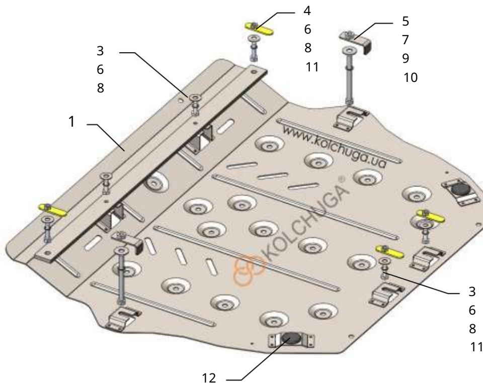
Schéma montáže.
