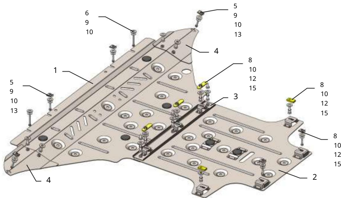
Schéma montáže ochrany motora a prevodovky
