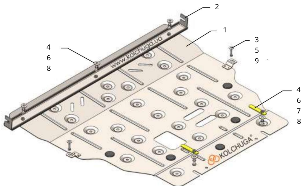
Schéma montáže.
