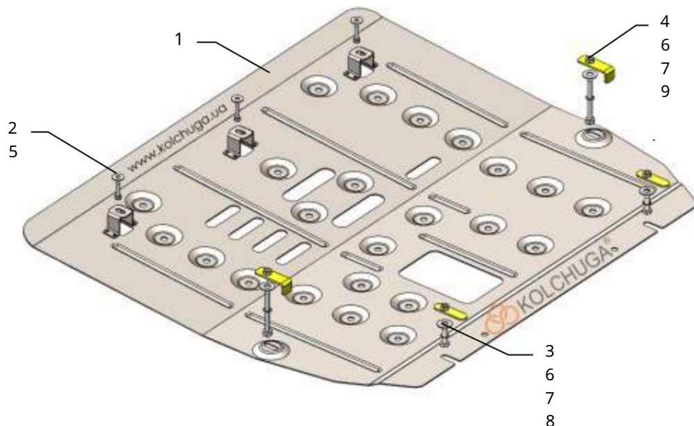
Schéma montáže.
