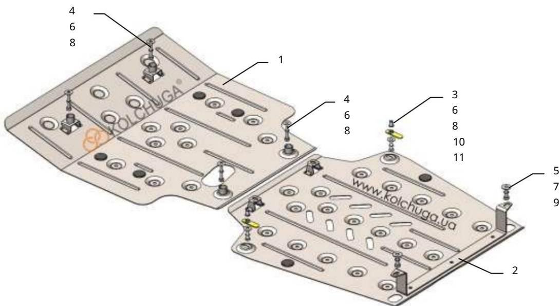
Schéma montáže.
