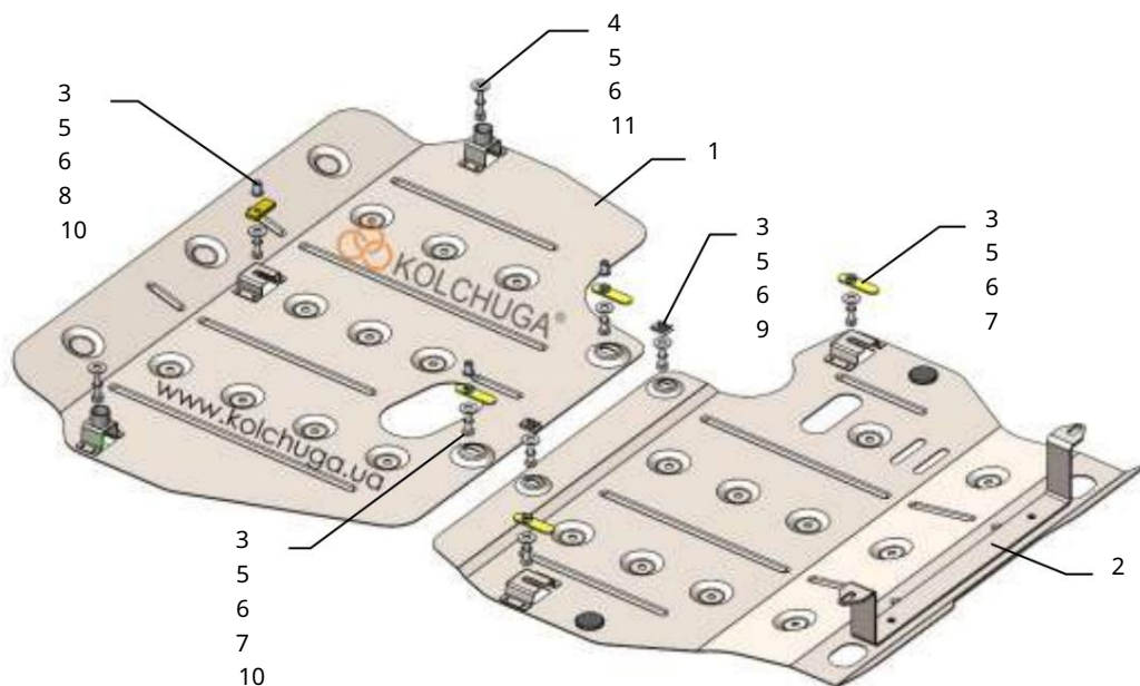
Schéma montáže.
