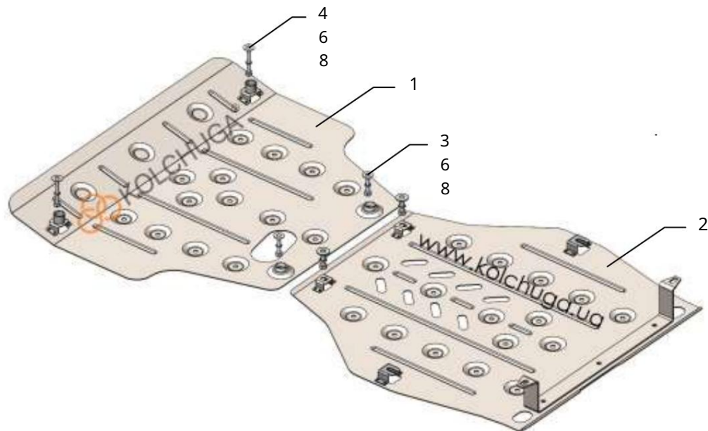
Schéma montáže.
