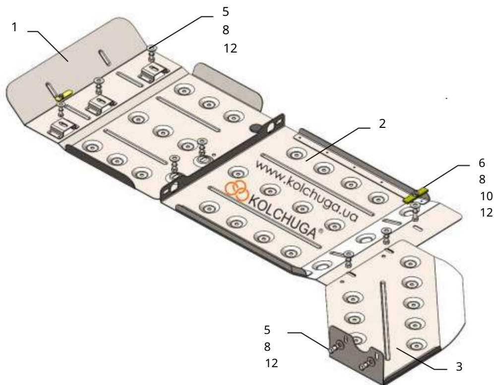
Schéma montáže.
