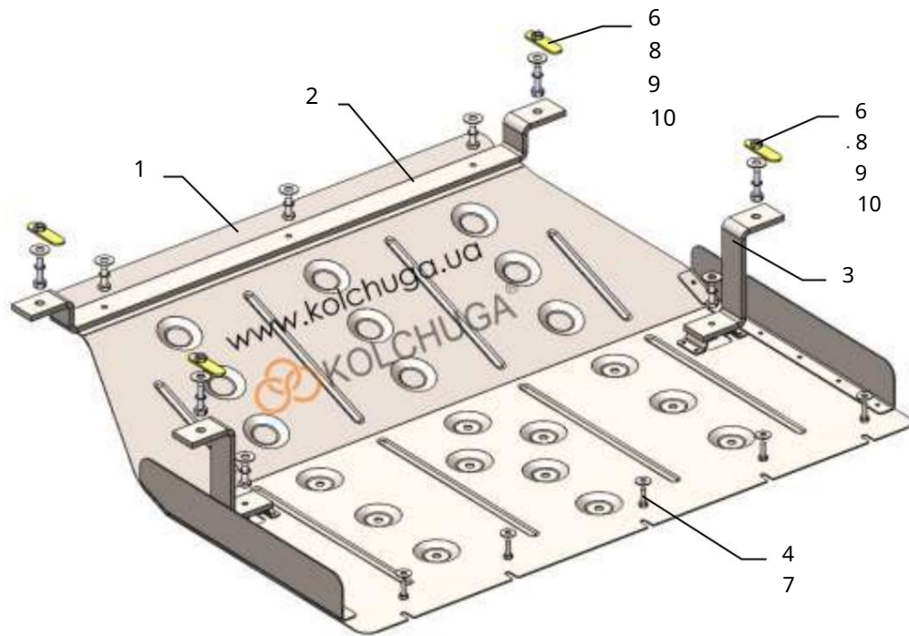
Schéma montáže.
