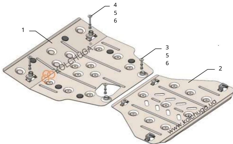
Schéma montáže.
