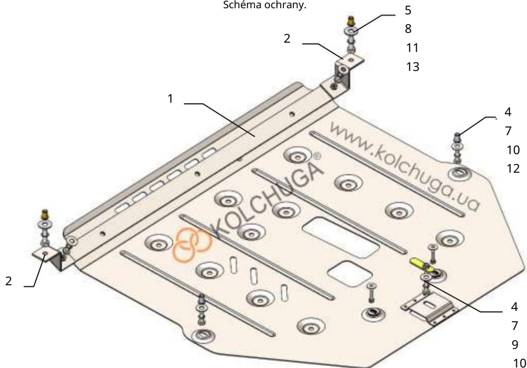
Schéma ochrany.
