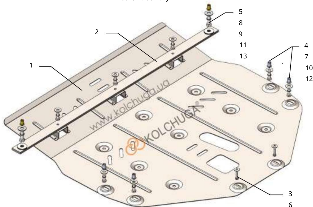
Schéma ochrany.
