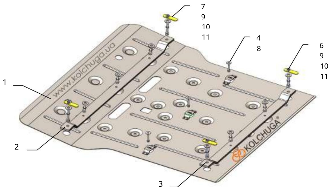
Schéma ochrany.
